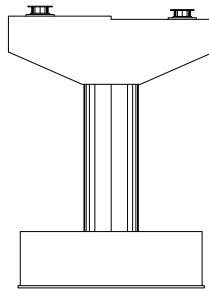
전면
